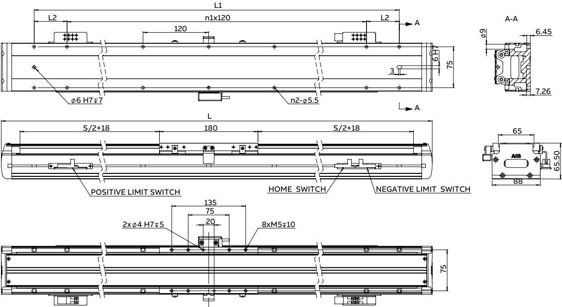
机械尺寸
