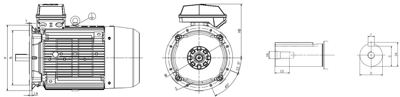
凸缘安装型电机 IM3001, B5 Flange-mounted motor IM3001, B5
